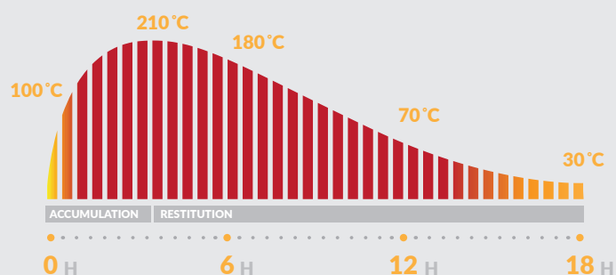
RÉPARTITION DE LA CHALEUR DANS LE TEMPS AVEC LE SYSTÈME DURASIC®
