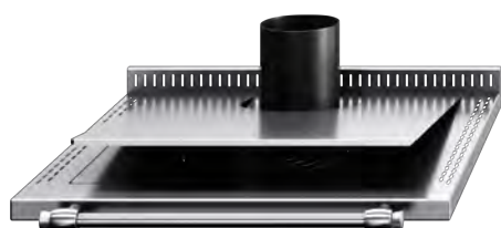
Couvercle avec découpe pour le passage du conduit
